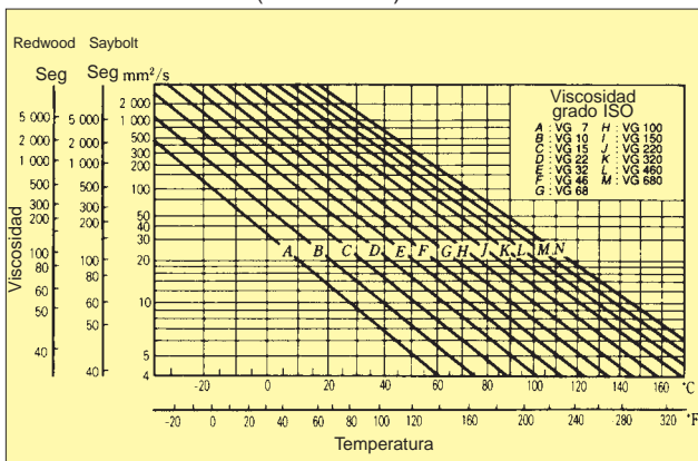
Ilustración 4.1 Relación entre viscosidad y temperatura
